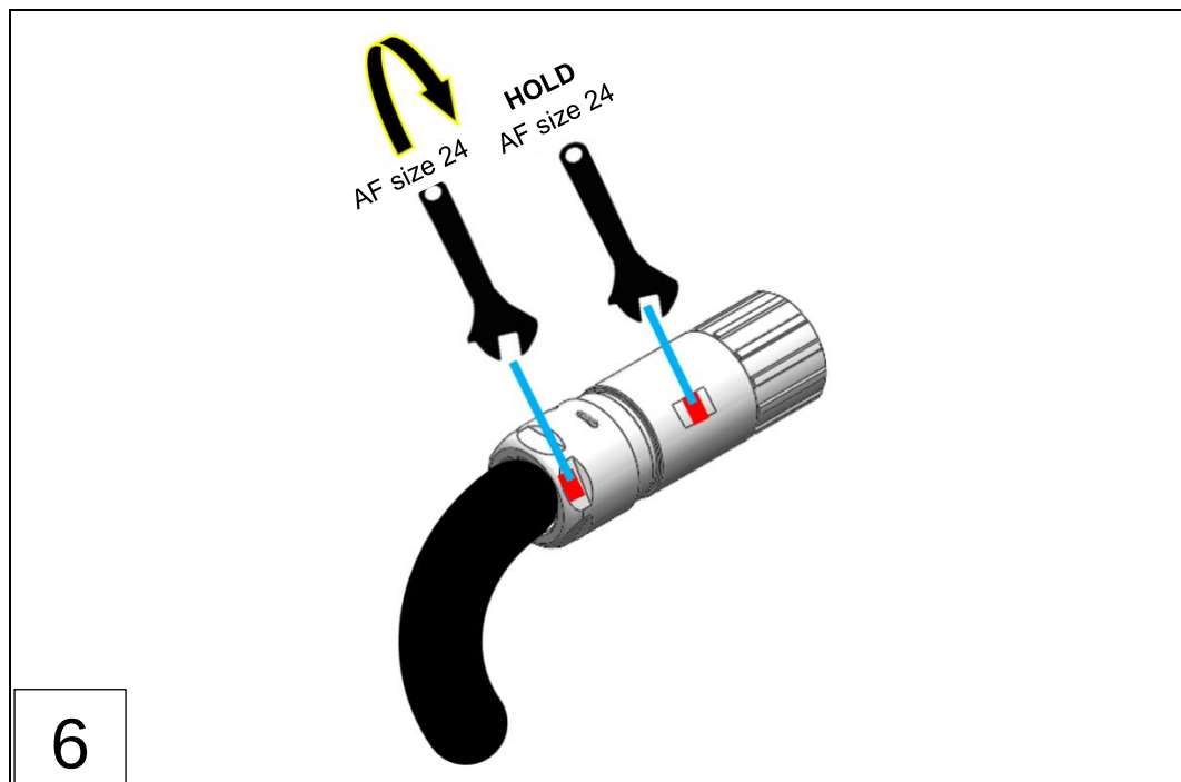
1: Cap nut
