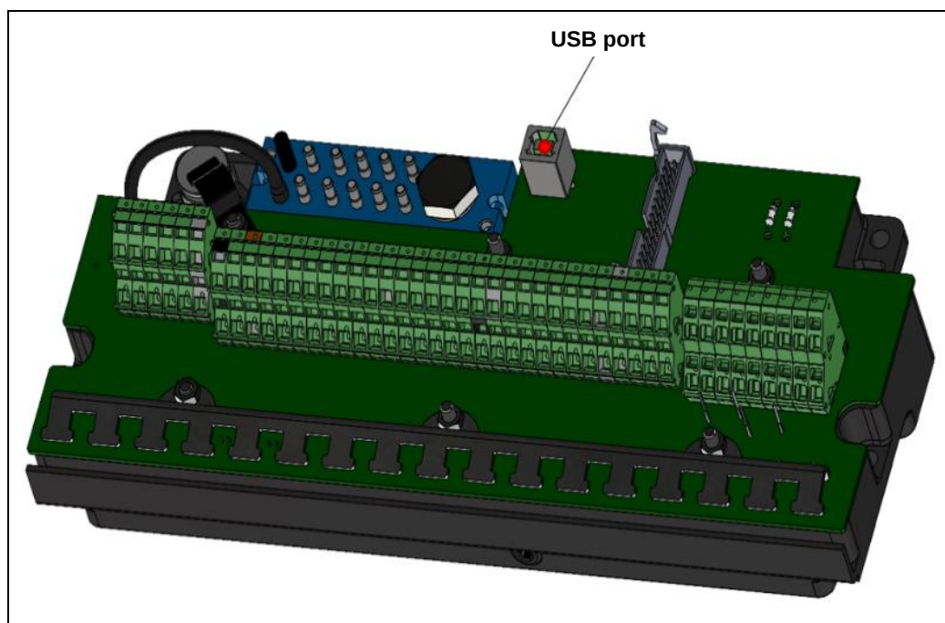
Fig.: 78 : VN301 plus central unit, USB port
