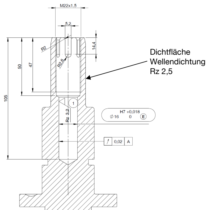
Abbildung 4: Sensor-Verbindung – Kurbelwellenadapter kurz (Beispiel)
