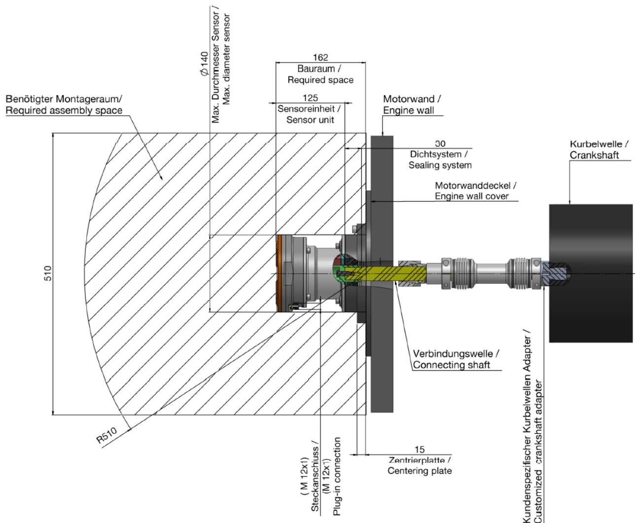
Abbildung 6: Sensorschnitt - lang (mit Wellendichtring)
