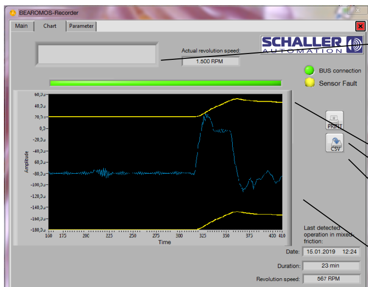
Abbildung 9: Graph- Ansicht
