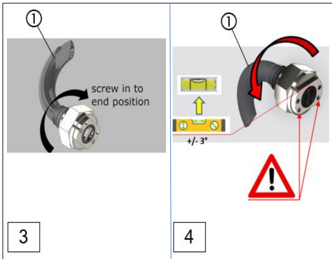
1: Ansaugkrümmer
